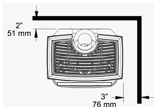
Figure 3. Dégagements d'installation parallèle.
